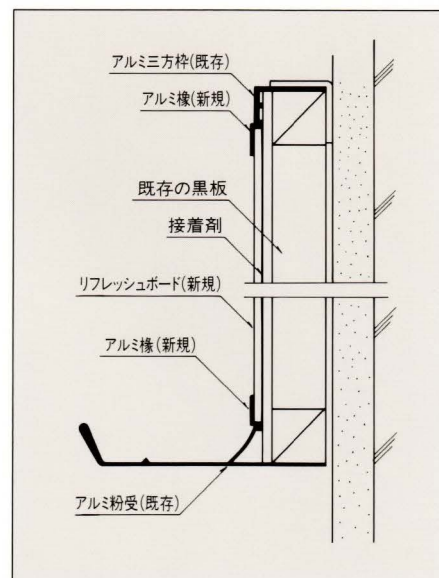
▲ アルミ枠付施工図
