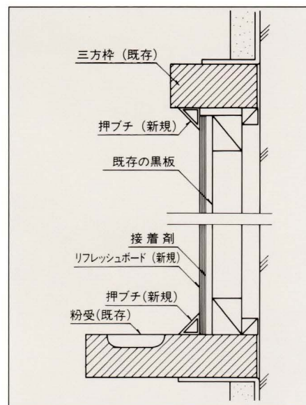
▲ 木枠付施工図
